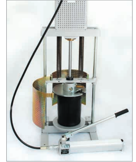
Hidrolik el pompalı versiyon
