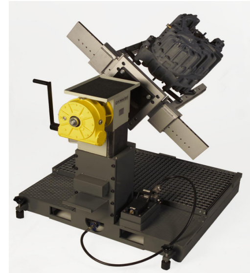
WW-GA1200 Üniversal Motor & Şanzıman Differansiyel Adaptörü
